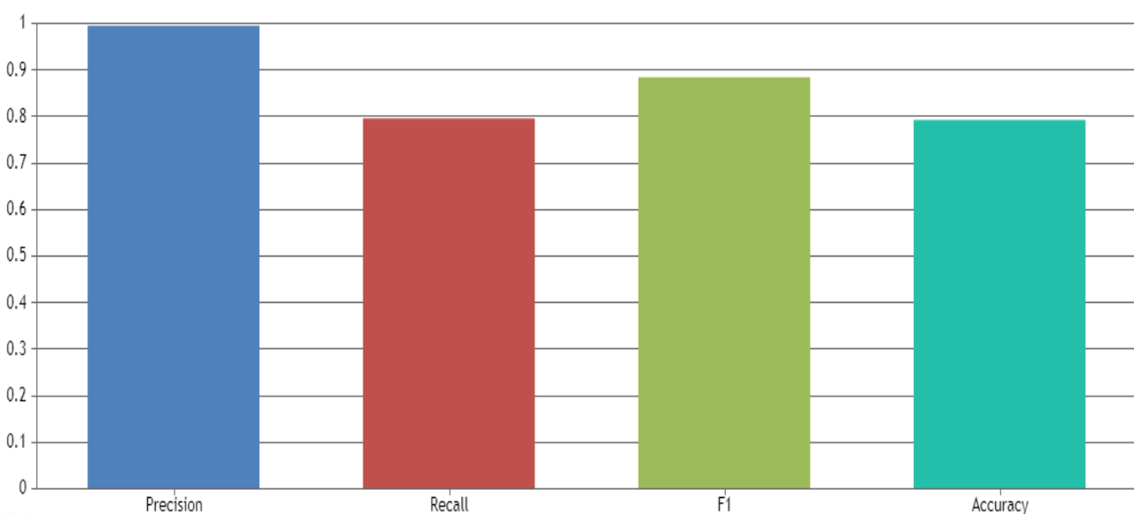
Fig. 3.SVM
