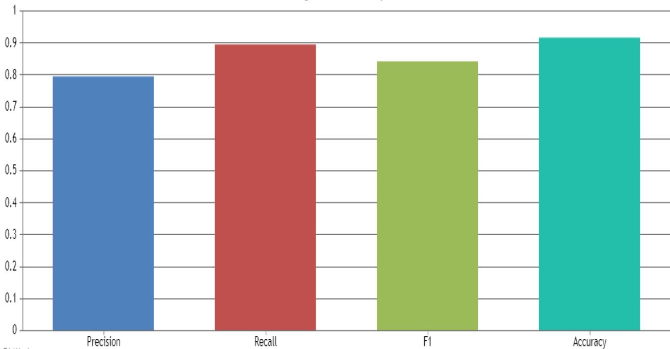
Fig. 7. Prism
