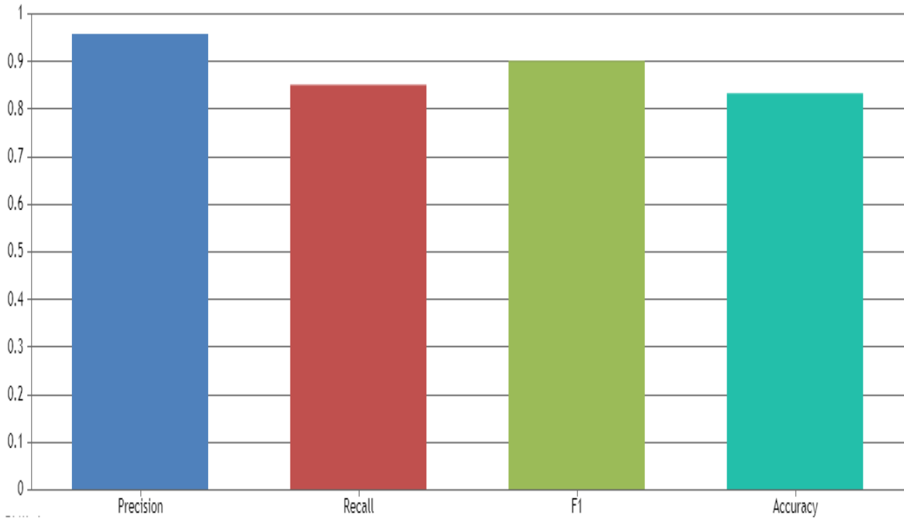
Fig. 6. Naïve Bayes
